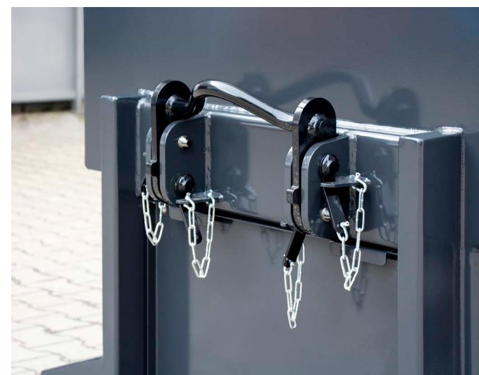
Abklappbarer und abnehmbarer Haken vorne
